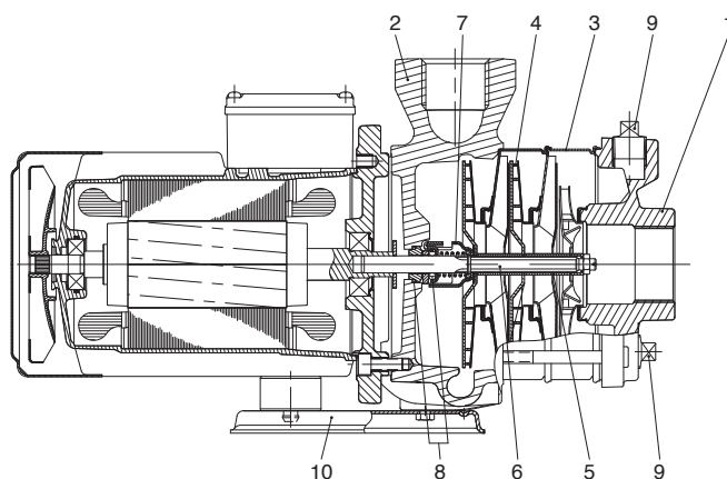
AB40x32, 40x40
