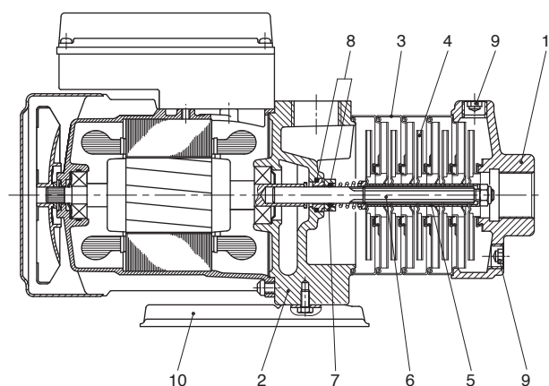
AB(I)25x25, 32x25
