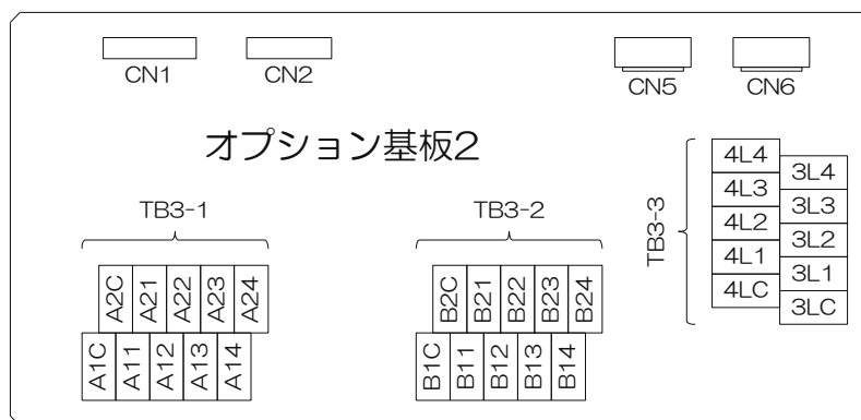
図 9-1 (b) オプション基板 2 詳細図
