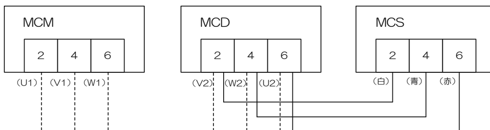
図 3-3-5(c) 電動機配線作業 2 (BN3S)
