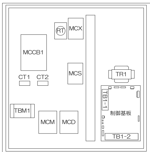
図 2-1-3(b) 制御盤の機器構成(スターデルタ起動 BN3S)
