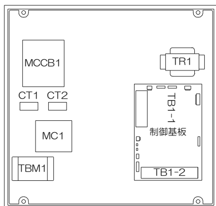
図 2-1-3(a) 制御盤の機器構成(直入起動 BN3L)
