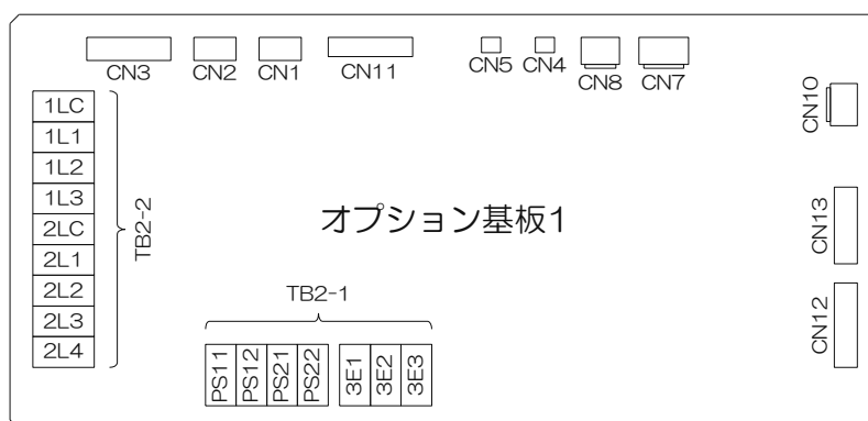
図 9-1 (a) オプション基板 1 詳細図
