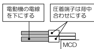
図 3-3-5(e) MCD への配線
