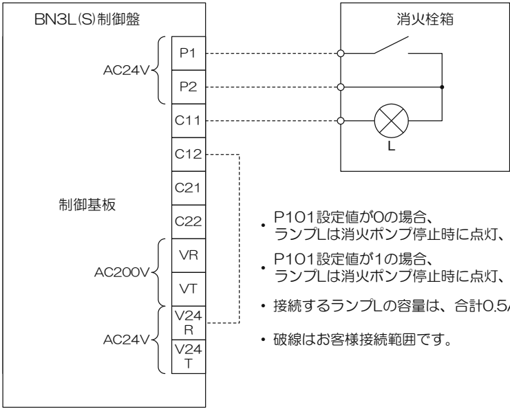
図 3-3-4(b) 消火栓箱接続例
