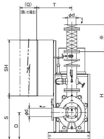
A-A矢視図
