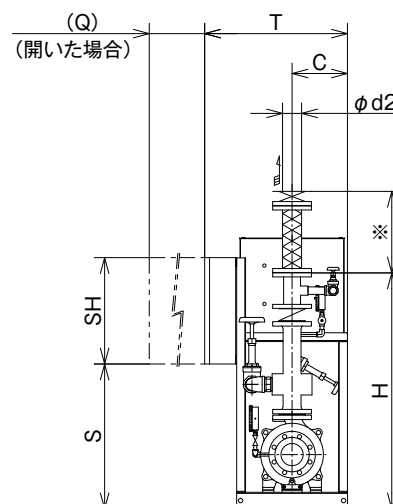
X-X矢視図
