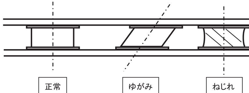
図 4 防振ゴム取付例
