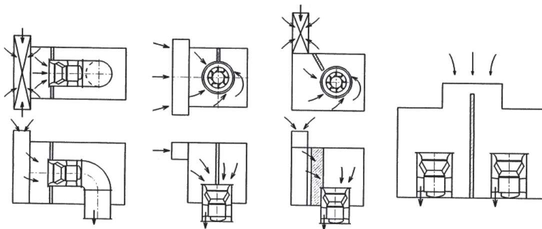
図8 吸込室の形状例
