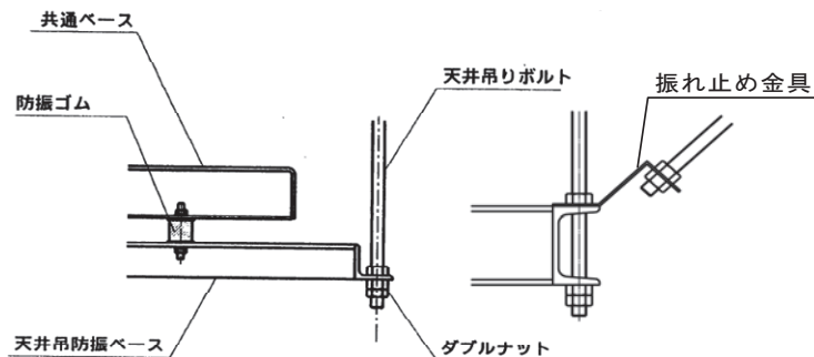
図 3 天井吊り取り付け例
