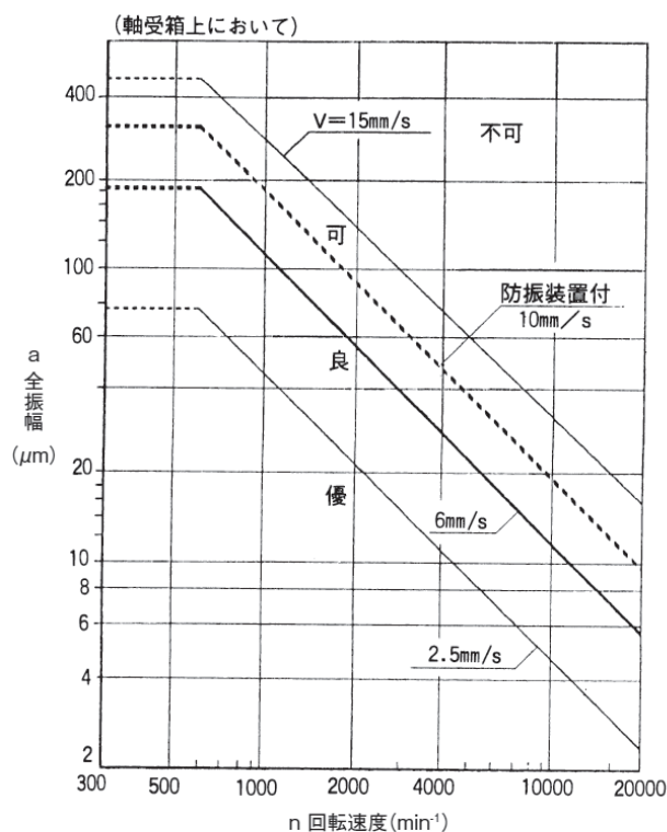
図 10 振動許容範囲
