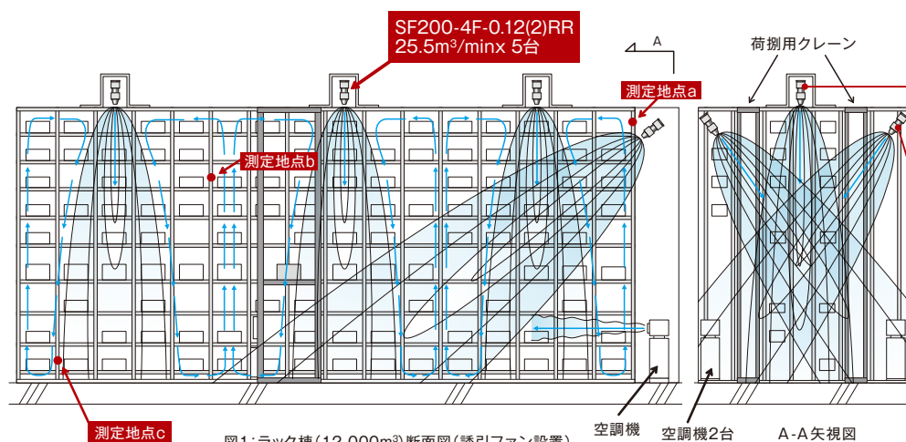
図1:ラック棟(12,000m³)断面図(誘引ファン設置)
