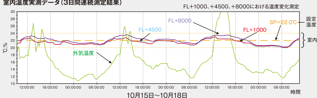
室内温度実測データ(3日間連続測定結果)
