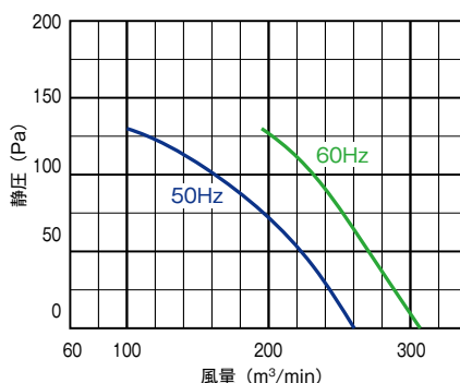
■羽根径 105cm/2200W-8P
