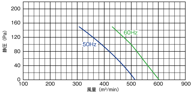
■羽根径 105cm/2200W-8P
