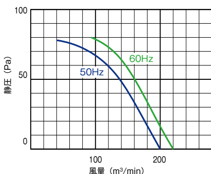
■羽根径 90cm/2200W-6P
