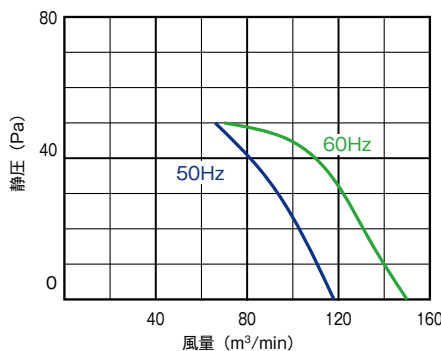
■羽根径 75cm/1500W-6P
