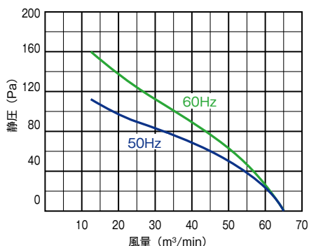
■羽根径 60cm/750W-6P
