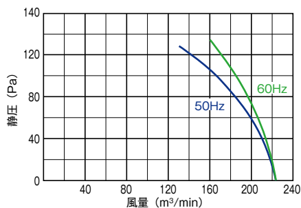
■羽根径 90cm/2200W-6P
