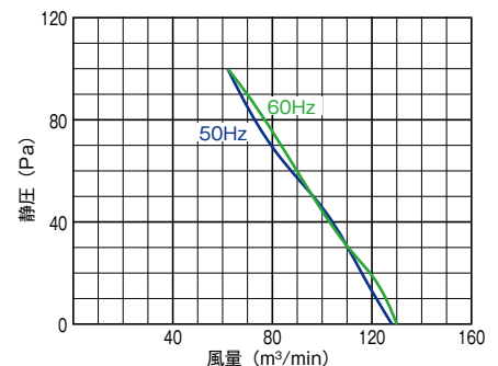
■羽根径 60cm/400W-8P
