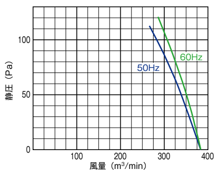
■羽根径 105cm/2200W-8P
