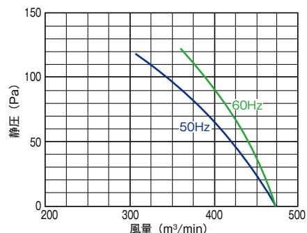
■羽根径 105cm/2200W-10P
