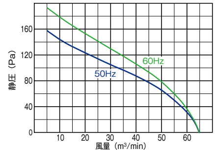
■羽根径 40cm/200W-4P
