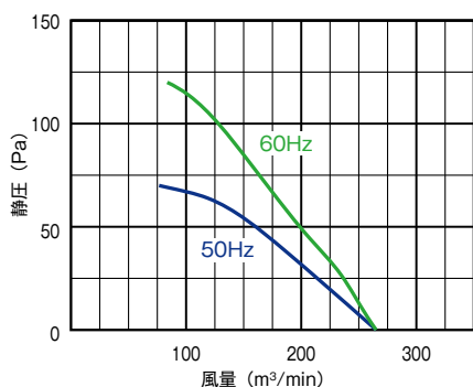
■羽根径 90cm/1500W-8P
