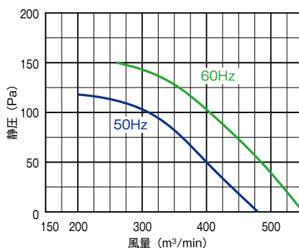
■羽根径 105cm/2200W-10P
