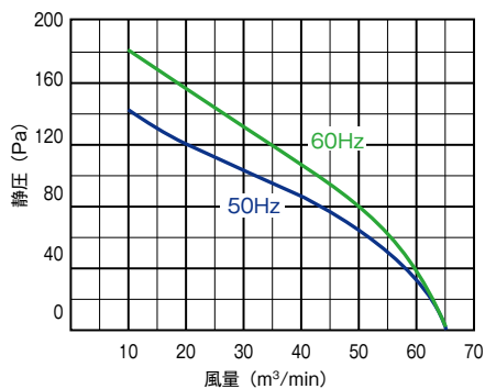
■羽根径 60cm/400W-8P
