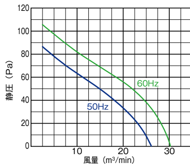
■羽根径 30cm/50W-4P
