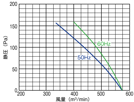
■羽根径 105cm/2200W-8P
