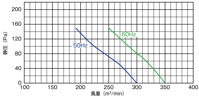
■羽根径 105cm/2200W-8P
