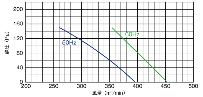
■羽根径 90cm/2200W-6P
