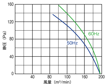
■羽根径 90cm/1500W-8P
