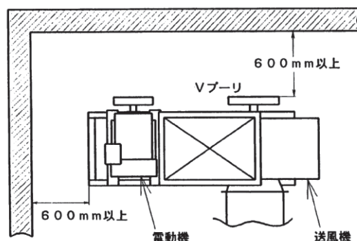
図 3 送風機の据付け(推奨)
