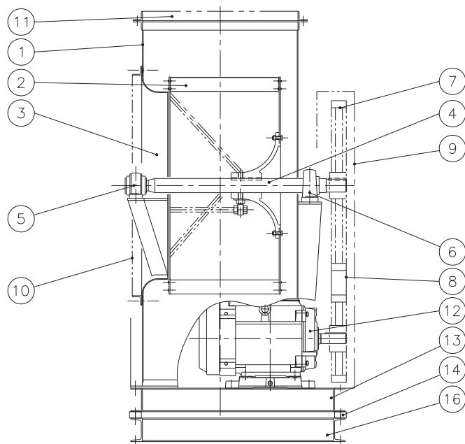
RS タイプ(CLF II (R)-RS 代表図)
