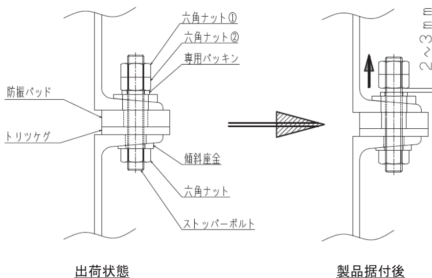
図 9 ストッパーボルト締結状態(防振パッド使用の場合)
