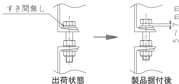
図 8 ストッパーボルト締結状態
