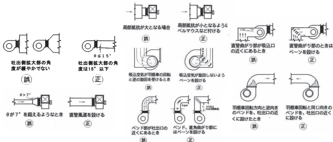
図 12 配管方法例
