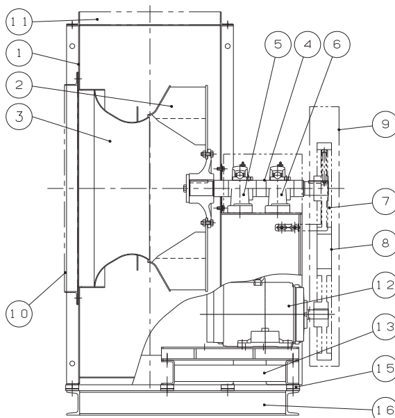
SOB タイプ(CMF3(R)-SOB 代表図)
