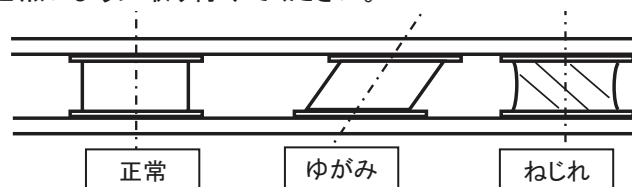
図 7 防振ゴム取付
