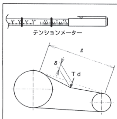
図 11 ベルトたわみ荷重測定法
